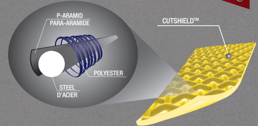
2 MICROSCOPIC VIEW OF A CUT SHIELD FIBRE APERÇU MICROSCOPIQUE D'UNE FIBRE CUT SHIELD
